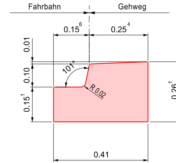
Ansicht Stirnseite links
