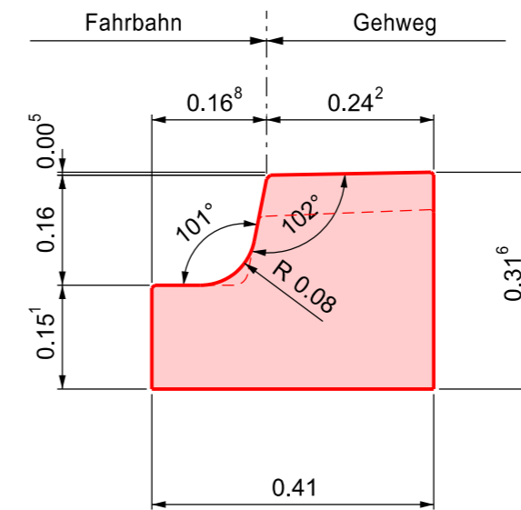
Ansicht Stirnseite links
