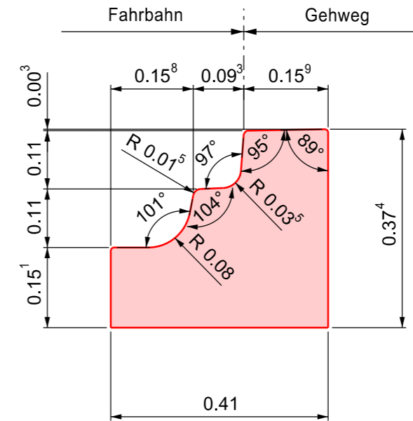
Ansicht Stirnseite links
