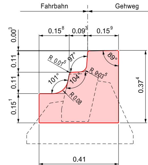
Ansicht Stirnseite links
