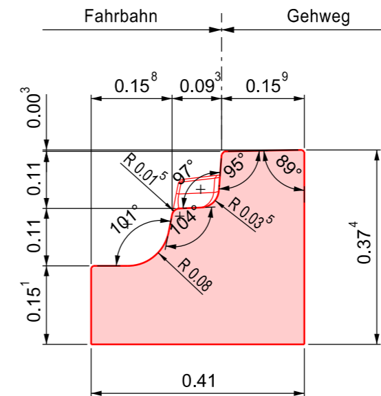
Ansicht Stirnseite links
