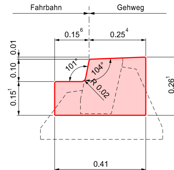
Ansicht Stirnseite links
